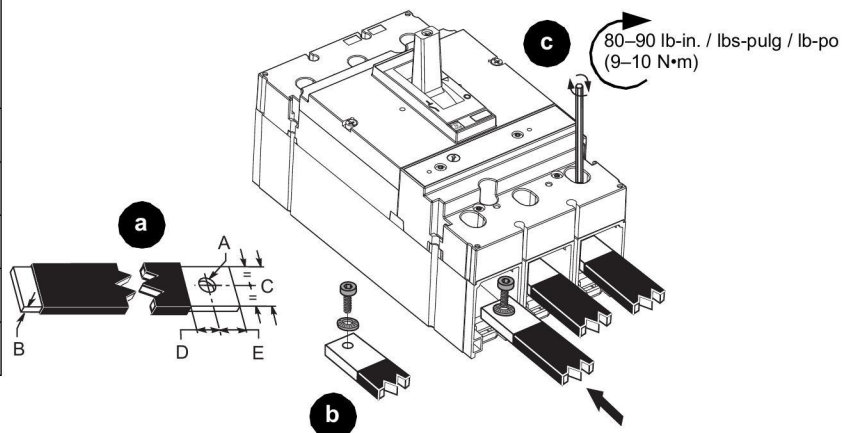
Figure / Figura / Figure / 图 6 : Bus and Bus Insulation Dimensions / Dimensiones de la barra y del aislamiento de la barra / Dimensiones de la barre-bus et de son isolation / 母排和母排绝缘尺寸
